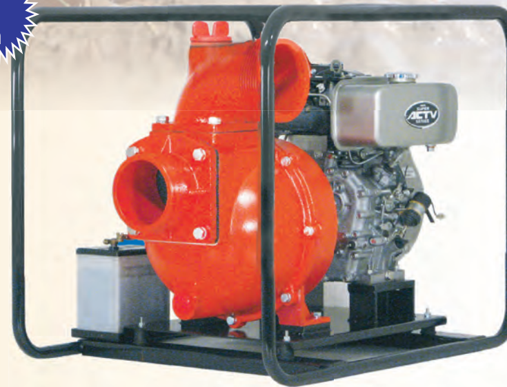
QP-602D (KUBOTA OC95) Max Head: 18m Max Flow: 2200ℓ/min
