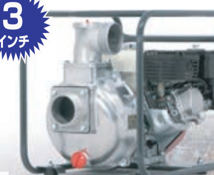
QP-305S (HONDA GX160) (MEiKi Power GB18G) 最大揚程: 70m 最大吐出量: 480ℓ/分
