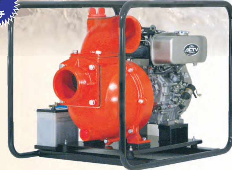
最大揚程: 18m 最大吐出量: 2200ℓ/分
