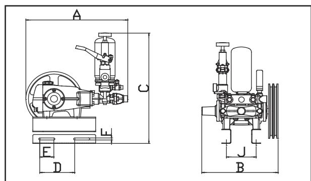
寸法 (mm)
