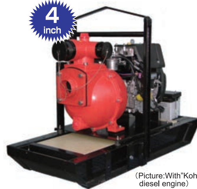
QP-T405SLTD (KUBOTA D722) Max Head: 95m Max Flow: 770ℓ/min
